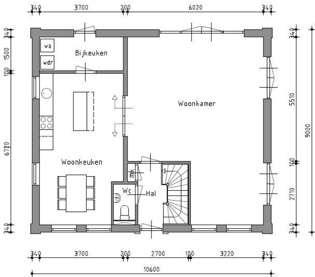
Begane grond
